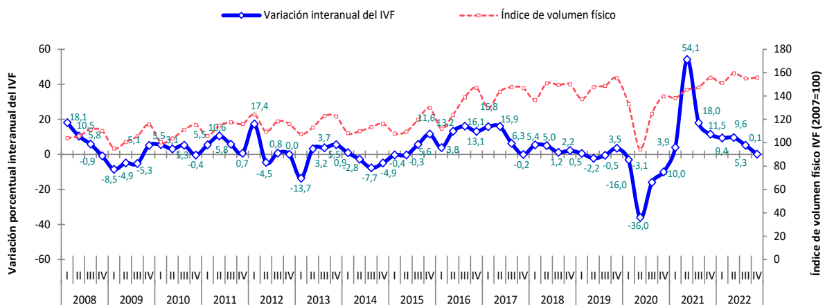
Gráfico N° 6 EXPORTACIONES DE BIENES Y SERVICIOS, 2008_I - 2022_IV (Valores a precios constantes de 2007)
