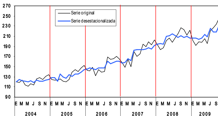
Índice mensual del Valor Agregado del Sector Construcción: 2004-2009
